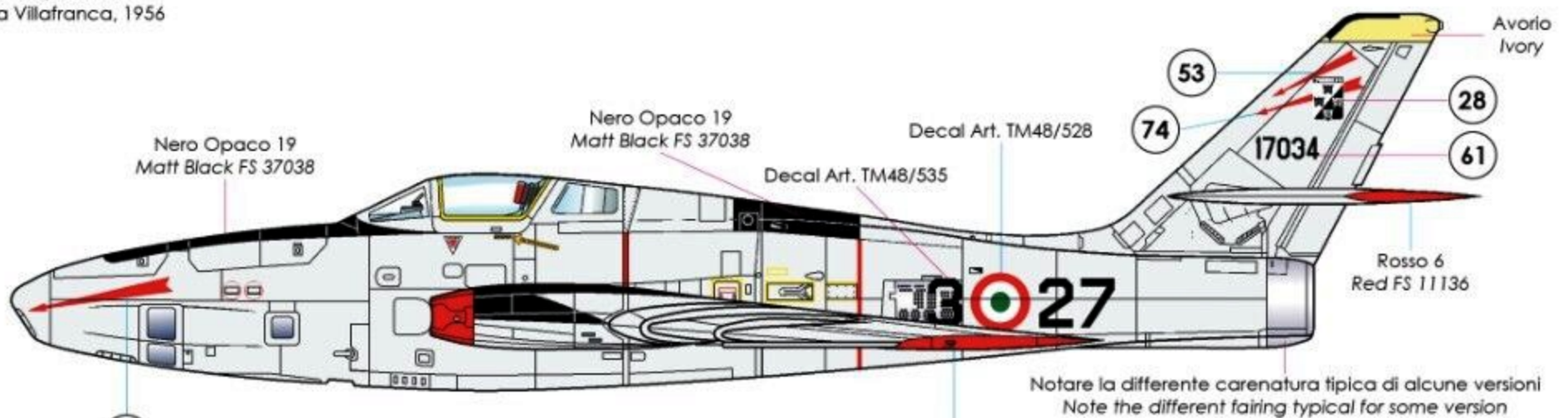
REPUBLIC RF-84F THUNDERFLASH SERIAL 51-7034 132° Gr., 3a Aer. Verona Villafranca, 1956
