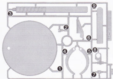
FB-1パーツ(クリア) (ABS)
